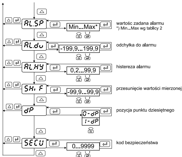
Rys. 5. Menu obsługi regulatora
