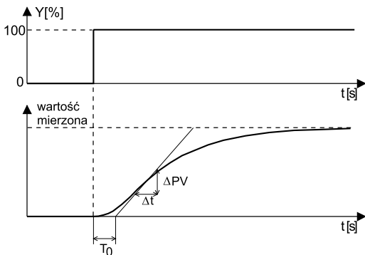
Rys. 10. Dobór nastaw metodą odpowiedzi na skok jednostkowy
