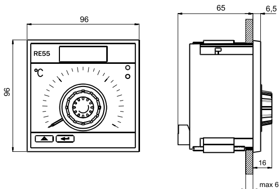
Rys. 2. Wymiary regulatora.
