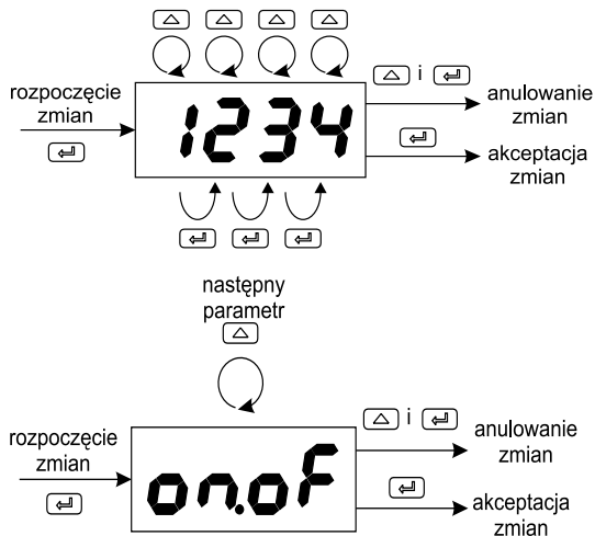
Rys. 7. Zmiana nastawy parametrów liczbowych i tekstowych.
