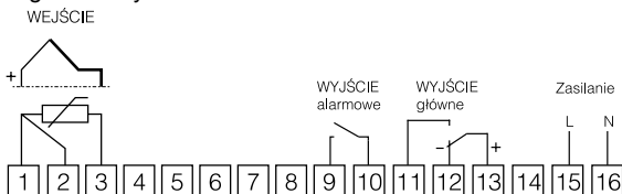
Rys. 3. Schemat podłączeń elektrycznych.
