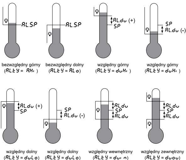
Rys. 9. Rodzaje alarmów.
