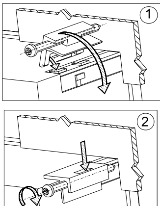
Rys. 1. Mocowanie regulatora.
